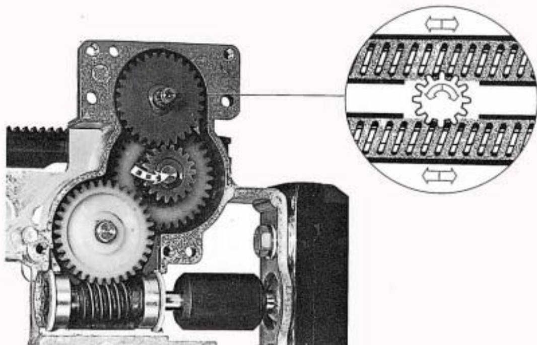
Dieses Zahnrad wurde mit dem Hebel herausgeschwenkt. Der Motor wird dadurch vom Antrieb getrennt.
